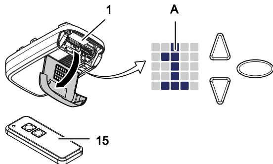
Abb. 4: Bedienelemente
