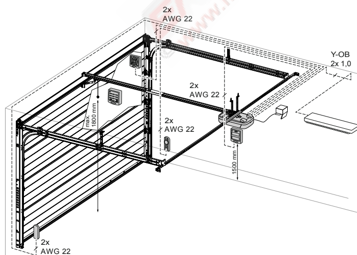
Abb. 3: Beispielinstallation Zubehör
