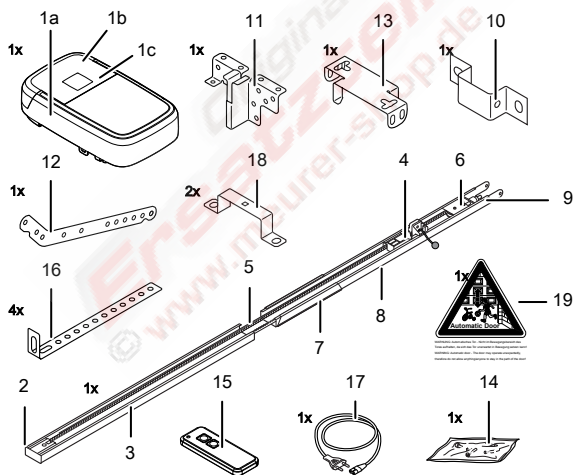
Abb. 2: Produktübersicht - Einzelteile
