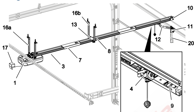
Abb. 1: Produktübersicht - Aufgebaut
