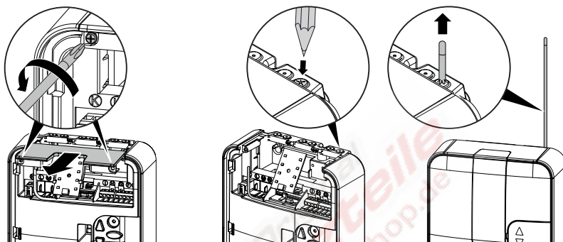
Abb. 8: Antenne verlegen
